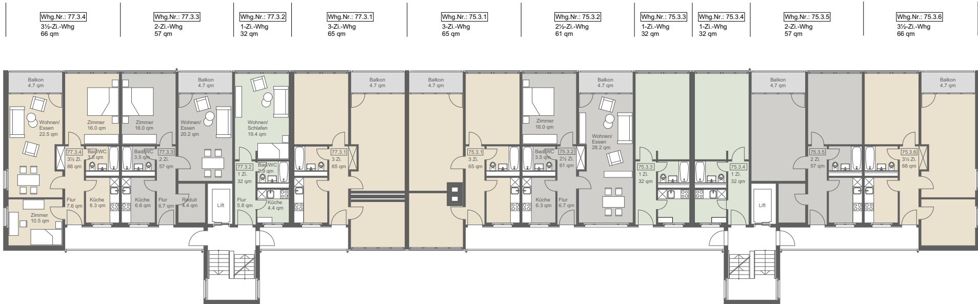
377 - 3.Obergeschoss
